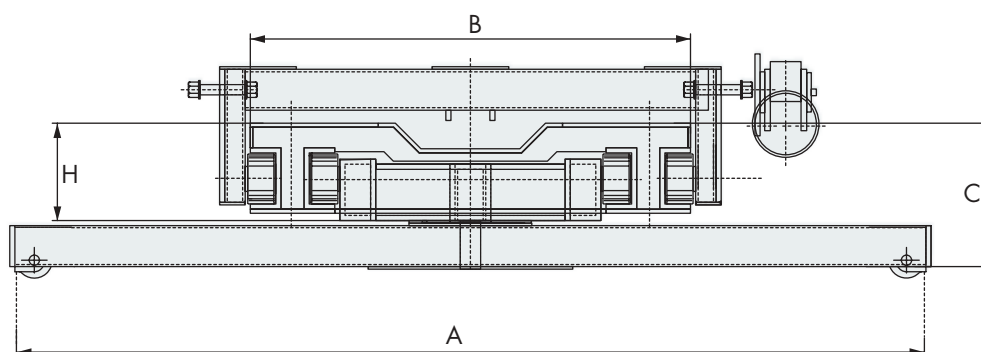
Trasloelevatore 400 Kg Codice 55P0000
